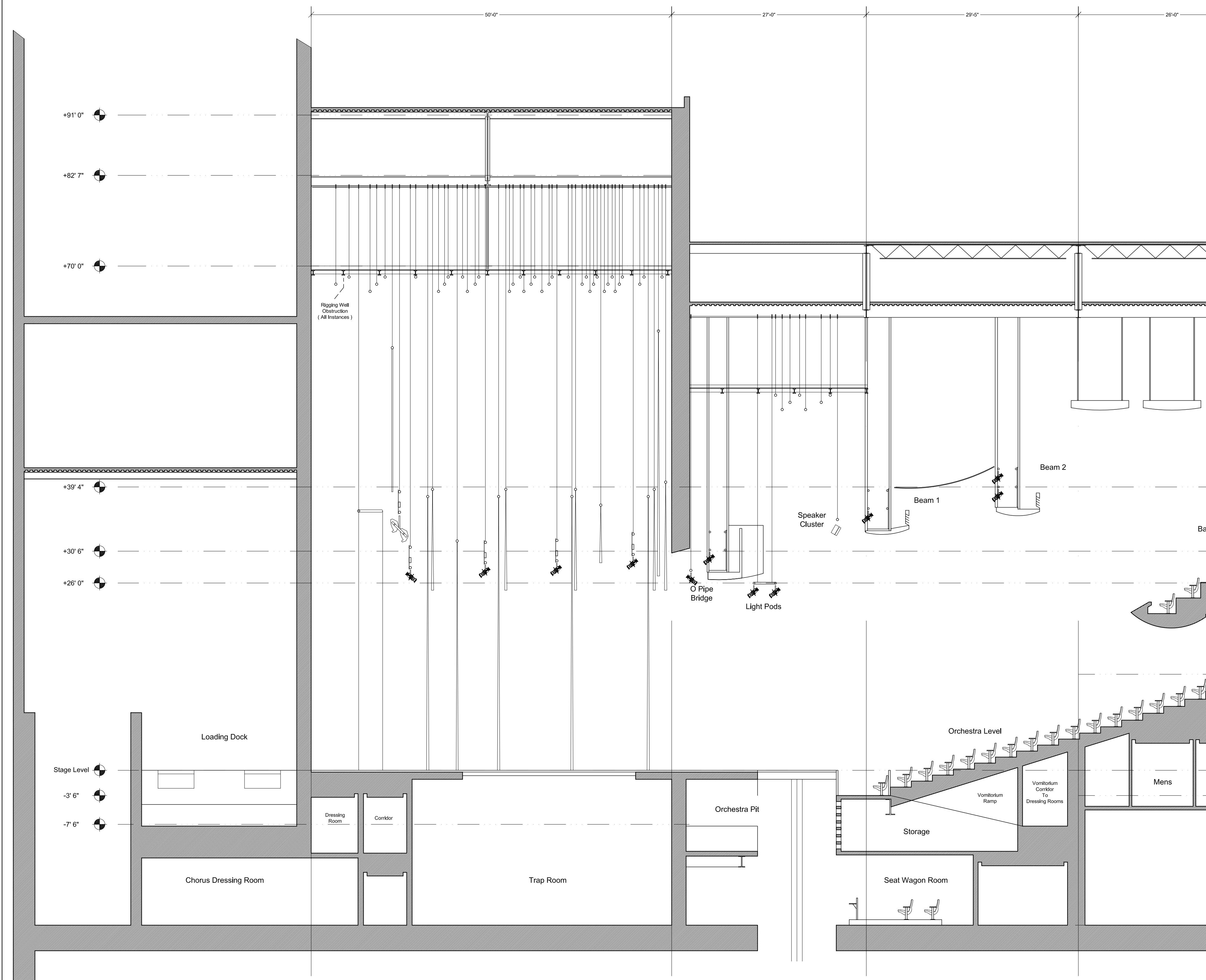
Polk Section Scale: 1/8" = 1' 0"
